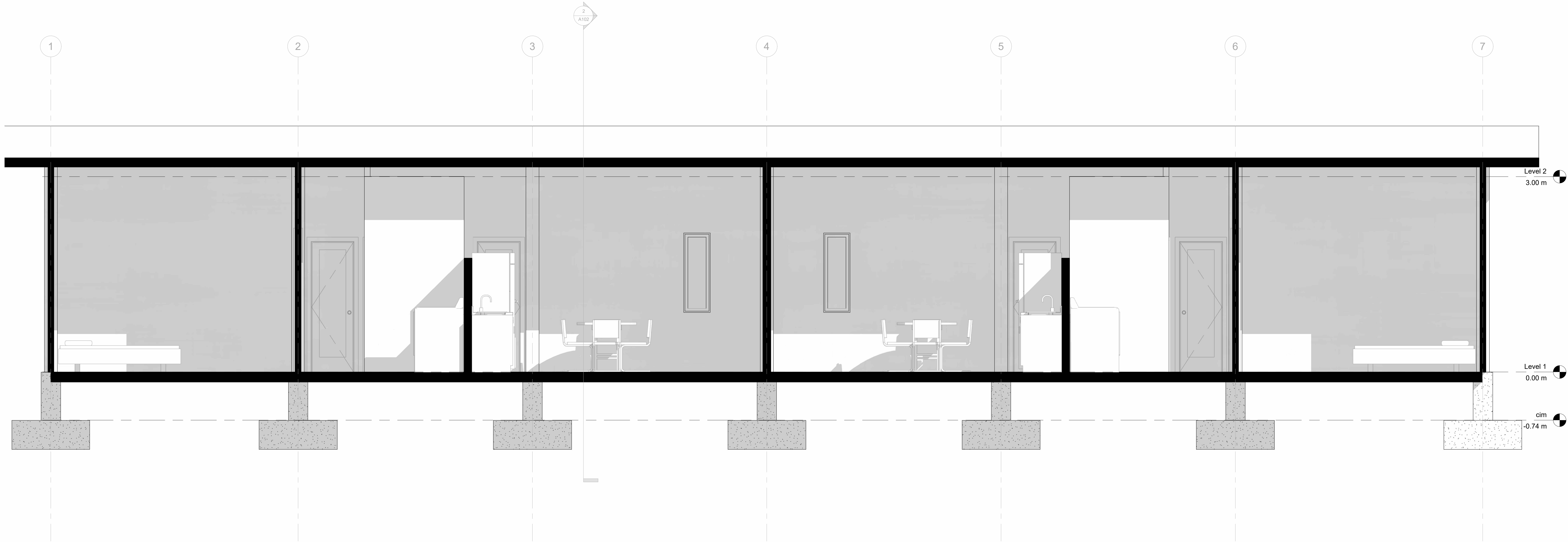
1 SECCIÓN 1 1 : 25
