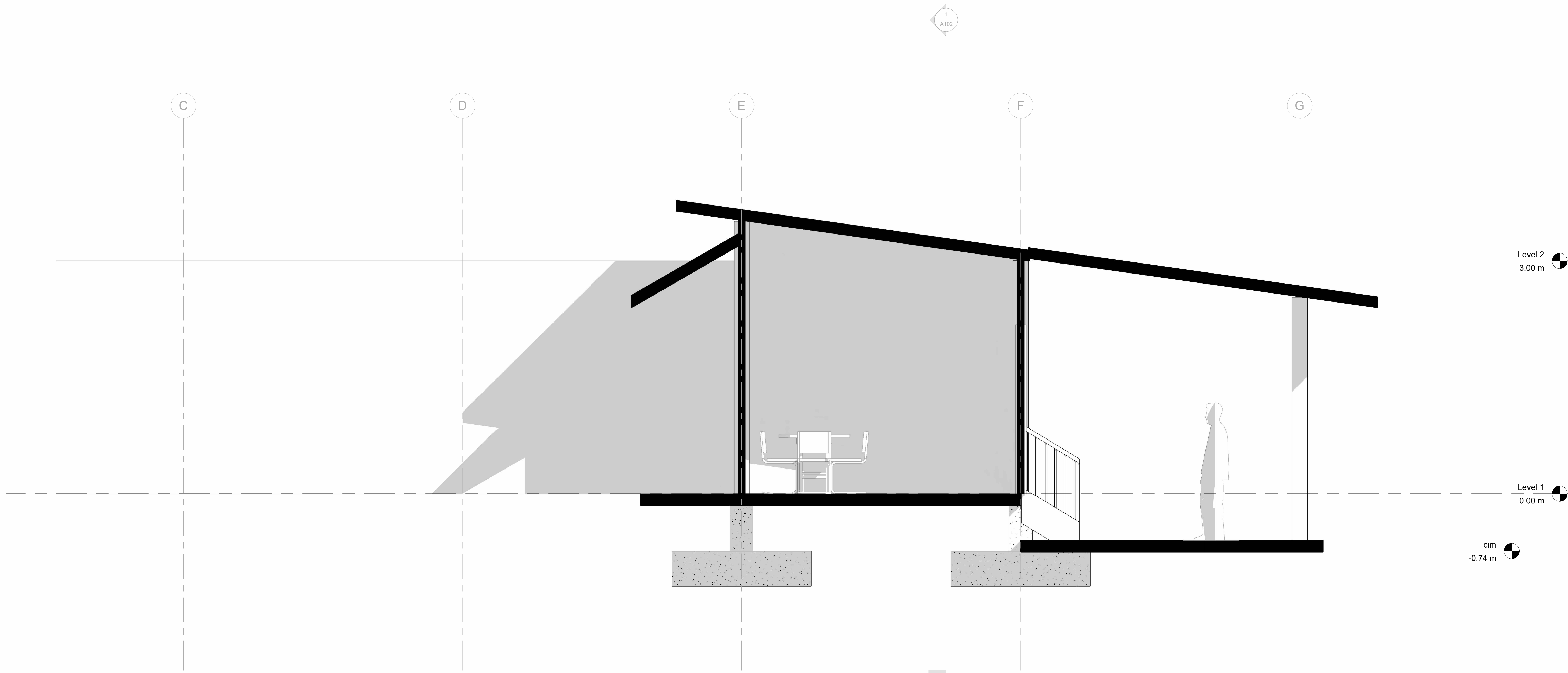
1 SECCIÓN 1 1 : 25
